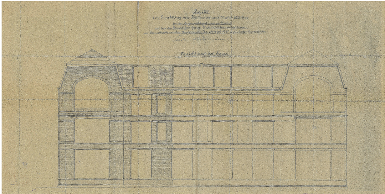
Nordansicht des Atelierhauses Siegmundshof 11. Landesarchiv Berlin
