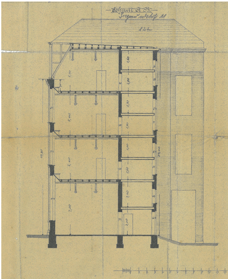
Seitlicher Aufriss des Atelierhauses Siegmundshof 11. Landesarchiv Berlin Raumhöhe bis 5.60 m.
